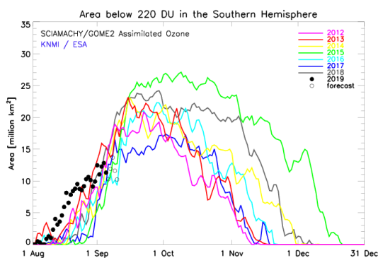
Figura 15b. El área de agujero de ozono para desde los años 1997 a 2018. El área de agujero de ozono es el área de la región donde el ozono total está por debajo de las 220 UD. Los datos son provistos por KNMI y están basados en los datos de los satélites GOME-2 y SCIAMACHY.
