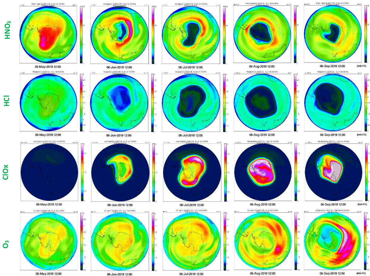
Figura 14. Resultados del modelo de asimilación BASCOE a 50 hPa. Este modelo se usa como parte del proyecto macc-II, ahora el NRT Análisis de ozono y especies relacionadas con el ozono ( http://macc.aeronomie.be/4_NRT_products/5_Browse_plots/1_Snapshot_maps/index.php?src=BASCOE&spc=o3&l=at-050hPa ). La primera fila (arriba) muestra la relación de mezcla del ácido nítrico (HNO 3 ). La segunda fila muestra la relación de mezcla para el ácido clorhídrico (HCl). La tercera fila, muestra la relación de mezcla para el óxido de cloro y su dímero (ClO x = ClO + 2Cl 2 O 2 ). La última fila (abajo) muestra la relación de mezcla del ozono.
