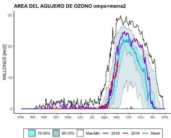
Figura 15a. Área (millones de km 2 ) donde la columna total de ozono es menos de 220 unidades Dobson. El año 2019 es mostrado en rojo (hasta el 6 de septiembre). El año 2018 se muestra en morado. La línea azul fuerte es el promedio de 1979-2018. El área sombreada azul opaca representa los percentiles 30 a 70 y el área sombreada en azul transparente representa los percentiles 10 a 90. El área de agujero de ozono el 3 de septiembre es 13.48 millón de km 2 . El gráfico está hecho en la SMN basado en datos descargados del sitio web de Vigilancia del ozono de la NASA, los cuales están basados en datos de NOAA/NCEP.
