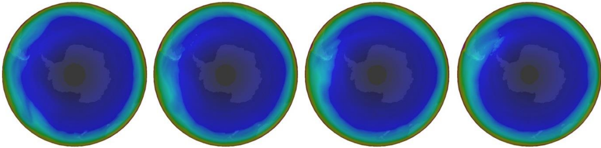
Figura 18. Mapas de proyección de la radiación UV para los días 7, 8, 9 y 10 de septiembre. Los mapas son tomados del Tropospheric Emission Monitoring Internet Service (TEMIS) – esa.
