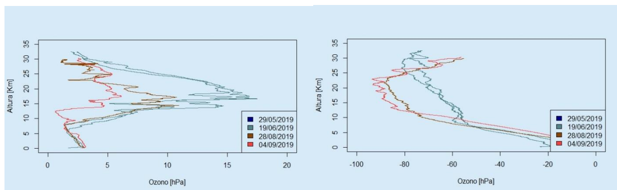
Figura 13. Se muestran los perfiles de cuatro días, los primeros dos, aún no presentan pérdida ozono, pero el último de la fila ya denota dicha pérdida.
