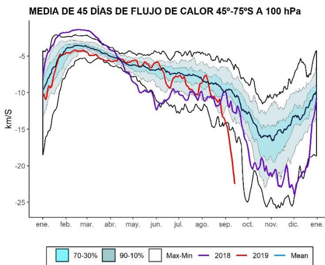
Figura 7. Serie de tiempo del flujo de calor meridional promediado sobre la región entre 45-75°S. La curva roja muestra los datos para 2019 (actualizado hasta el 20 de Agosto). Note que un gran número negativo significa un gran flujo de calor. Los valores cercanos a cero significan un flujo de calor pequeño. La línea azul oscura respresenta la media para el periodo 1979-2018. Las líneas externas negras, son los máximos y mínimos durante el periodo 1979 – 2018. Las líneas sombreadas en azul de adentro hacia afuera, son los percentiles de 70 – 30% y de 10 – 90%, finalmente la línea morada representa al año 2018.
