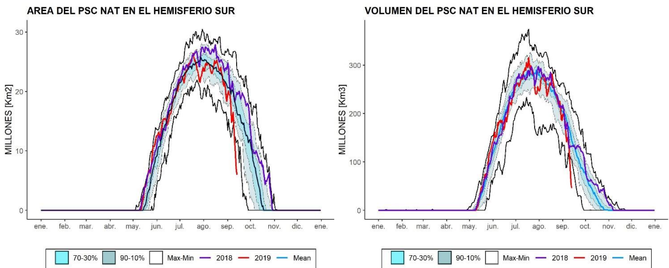
Figura 5 y 6. Serie de tiempo del Área y volumen de las nubes estratosféricas polares (NAT), sobre la región Antártica, donde la temperatura está suficientemente baja para la formación de ácido nítrico trihidratado (NET tipo I) en el nivel isentrópico de 460 K. La línea color roja representa la evolución del tamaño y volumen de la PSC NAT para el año 2019, la línea morada representa el mismo parámetro para el año 2018, la línea azul oscura representa la media para el periodo 1979-2018. Las líneas externas negras, son los máximos y mínimos históricos durante el periodo 1979 – 2018. Las líneas sombreadas en azul de adentro hacia afuera, son los percentiles de 70 – 30% y de 10 – 90%.
