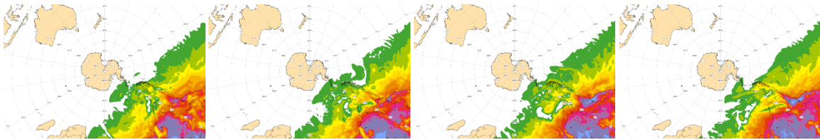
Figura 19. Mapas de proyección de la radiación UV para los días 7, 8, 9 y 10 de septiembre. Los mapas son tomados del Copernicus Atmosphere Monitoring Service (CAMS) UV index forecasts.
