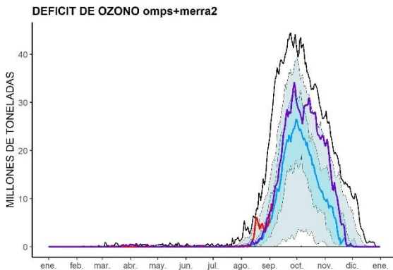
Figura 16a. Déficit de masa de ozono para 2019 (curva roja). La línea color morado, representa el año 2018. La línea azul fuerte es la media del periodo 1979-2018. Las líneas sombreadas en azul es el percentil de 30% y 70%, mientras que las líneas sombreadas con azul claro y transparente es el percentil de 10% y 90%. Finalmente, las líneas externas en negro son los máximos y mínimos históricos del periodo 1979 – 2018. Este gráfico es producido por el SMN basado en datos descargados del sitio web de Vigilancia del ozono de la NASA, los cuales están basados en datos
