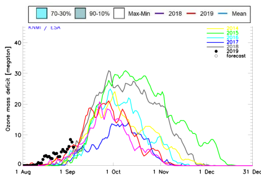
Figura 16b. Déficit de masa de ozono para 2019 (curva y puntos negros (pronóstico de 5 días). Algunos otros años seleccionados con una baja sustancial de ozono se muestran para ser comparados.. Los círculos abiertos representan el pronóstico para los siguientes cinco días. La línea gris gruesa es la media de 1979-2018. Este gráfico es producido por la OMM y está basado en datos del sitio web del TEMIS del KNMI.
