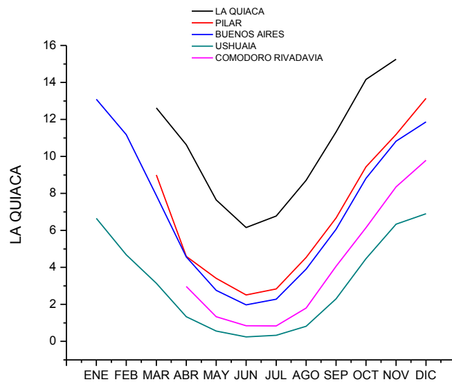
Figura 17. Promedio mensual del índice UV máximo diario para todos los lugares donde se tiene la suficiente cantidad de datos.
