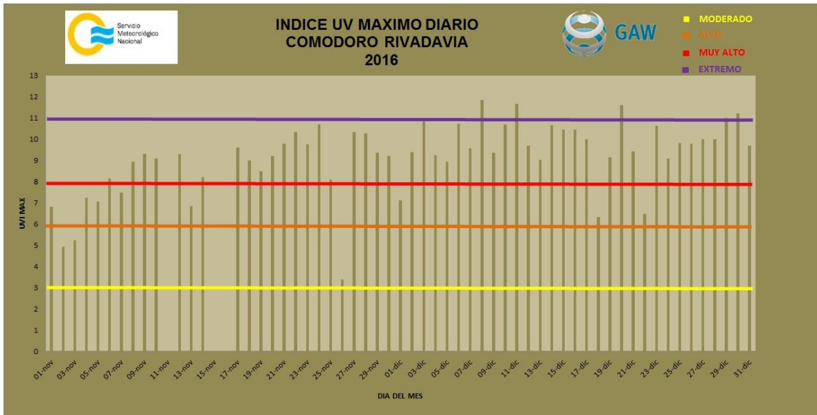
Figura 5. Índice UV máximo diario medido en Comodoro Rivadavia.
