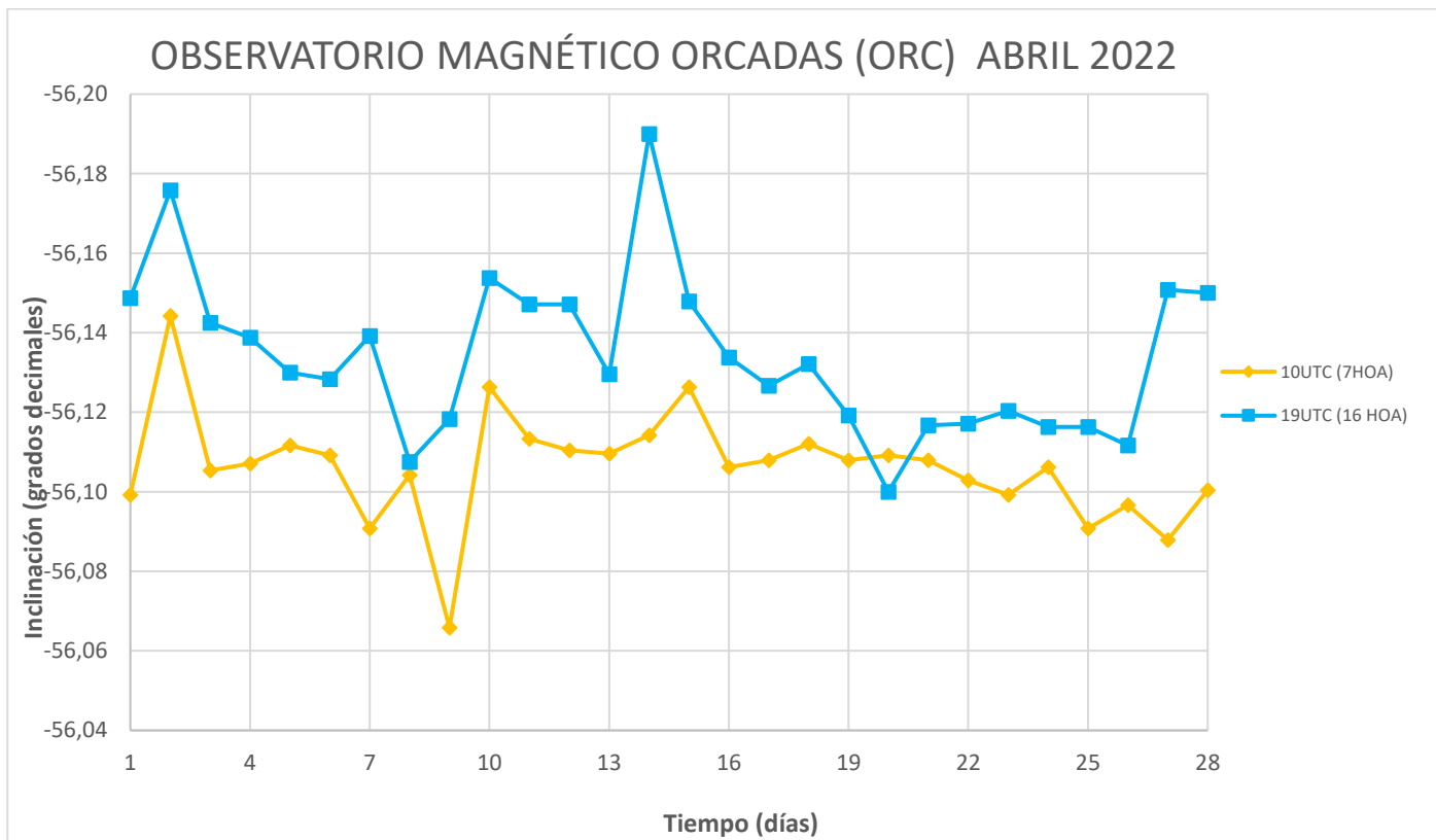
Figura 6: Inclínación magnética en función del tiempo
