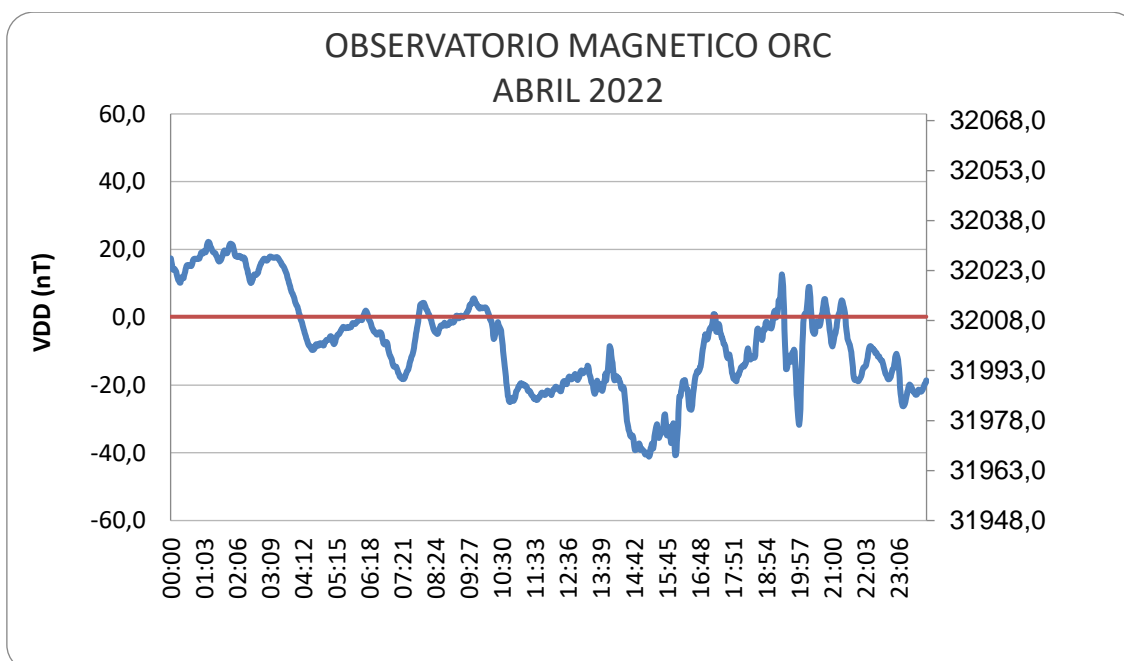
Figura 9: Variación Diaria Perturbada del mes de abril
