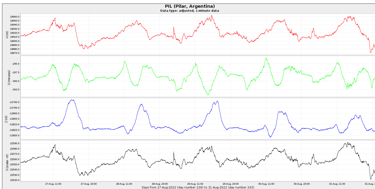
Figura 4c: Componentes del campo magnético del 22 al 31 de agosto. En rojo se ve la componente horizontal (H) y en azul la vertical (Z), ambas en nT. En verde se presenta la declinación del campo magnético (D) en minutos y en negro la intensidad del campo magnético en nT.
