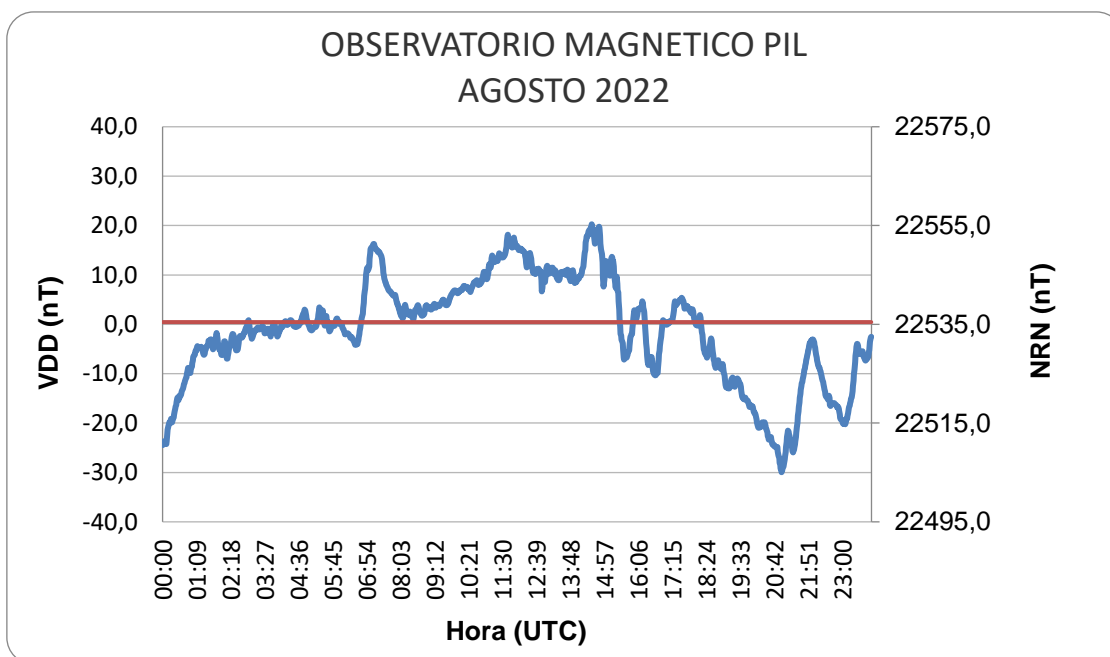
Figura 9: Variación Diaria Perturbada del mes de agosto
