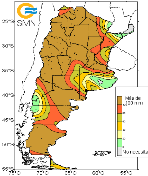
Agua necesaria para no estar en Sequía en los próximos 10 días a partir del 10 de diciembre de 2022
