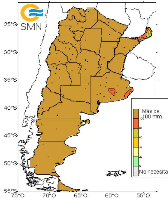
Agua necesaria para comenzar a tener Excesos en los próximos 10 días a partir del 10 de diciembre de 2022
