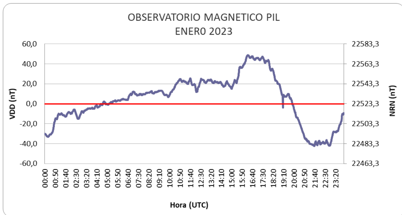
Figura 9: Variación Diaria Perturbada del mes de enero
