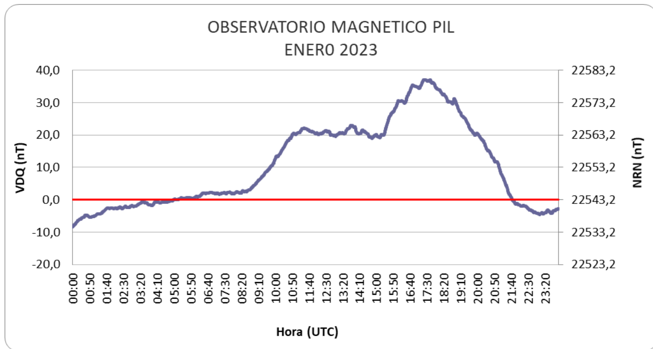
Figura 8: Variación Diaria Calma del mes de enero
