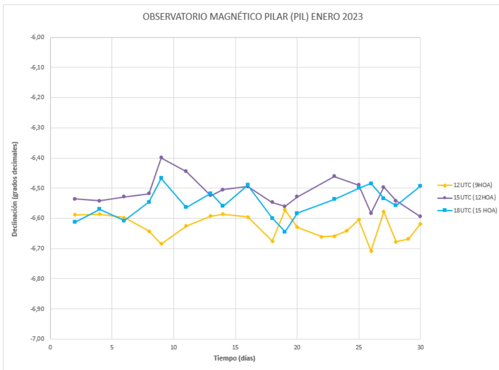
Figura 5: Declinación magnética en función del tiempo
