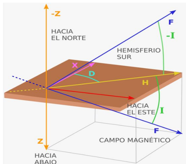
Figura SEQ Figura \* ARABIC 3: Componentes del campo magnético
