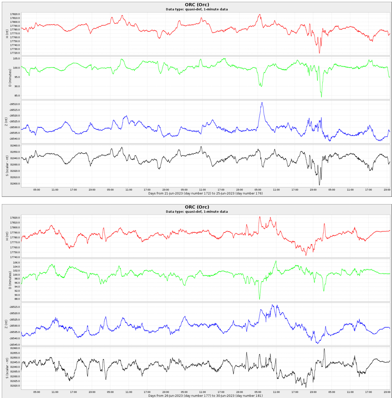
Figura 4c: Componentes del campo magnético del 21 al 30 de junio. En rojo se ve la componente horizontal (H) y en azul la vertical (Z), ambas en nT. En verde se presenta la declinación del campo magnético (D) en minutos y en negro la intensidad del campo magnético en nT.
