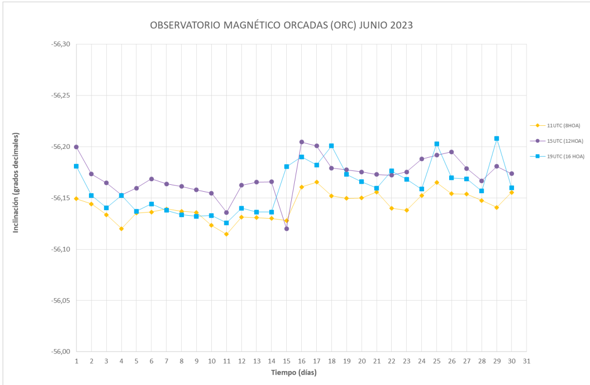
Figura 6: Inclínación magnética en función del tiempo
