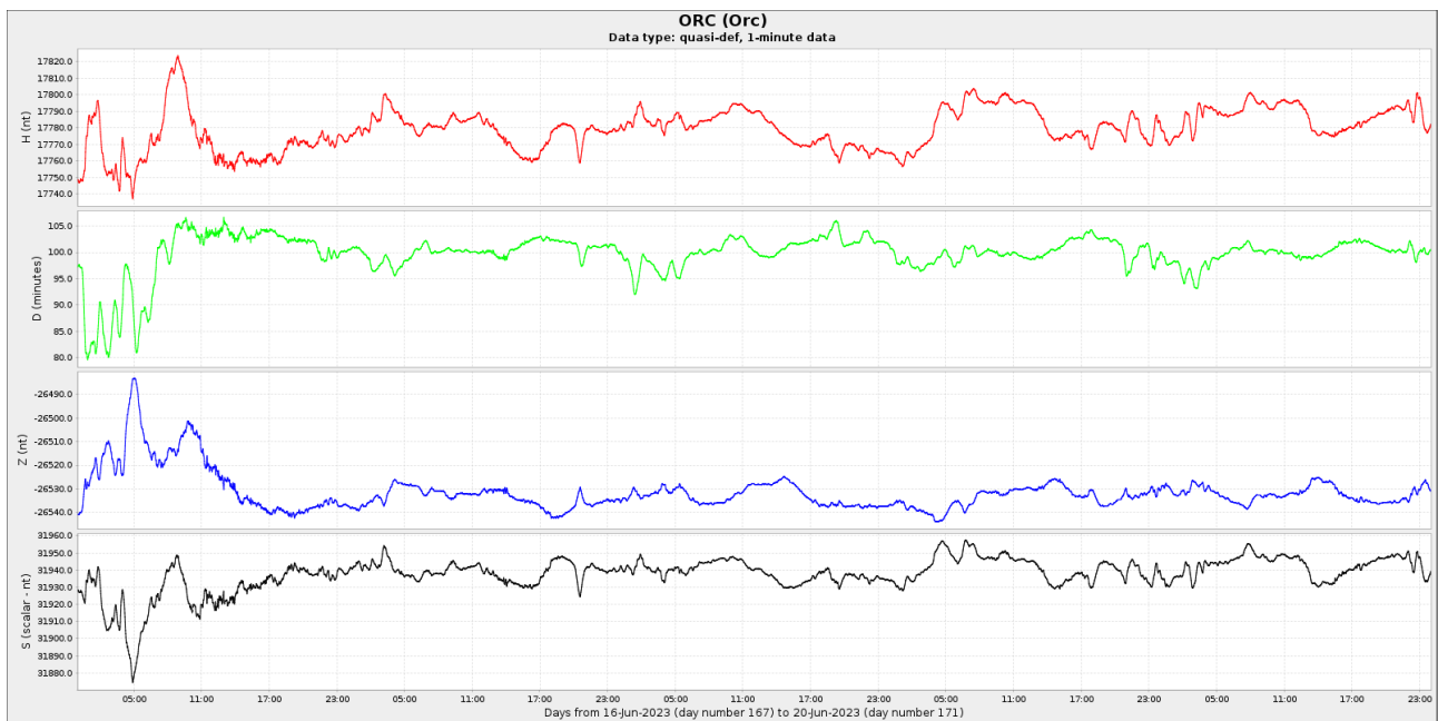
Figura 4b Componentes del campo magnético del 11 al 20 de junio. En rojo se ve la componente horizontal (H) y en azul la vertical (Z), ambas en nT. En verde se presenta la declinación del campo magnético (D) en minutos y en negro la intensidad del campo magnético en nT.
