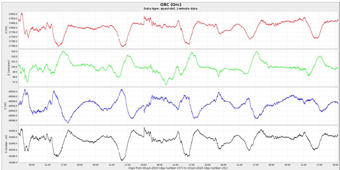
Figura 4a: Componentes del campo magnético del 1 al 10 de junio. En rojo se ve la componente horizontal (H) y en azul la vertical (Z), ambas en nT. En verde se presenta la declinación del campo magnético (D) en minutos y en negro la intensidad del campo magnético en nT
