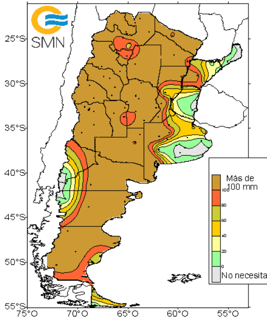
Agua necesaria para tener Buenas Condiciones en los próximos 10 días a partir del 31 de julio de 2023
