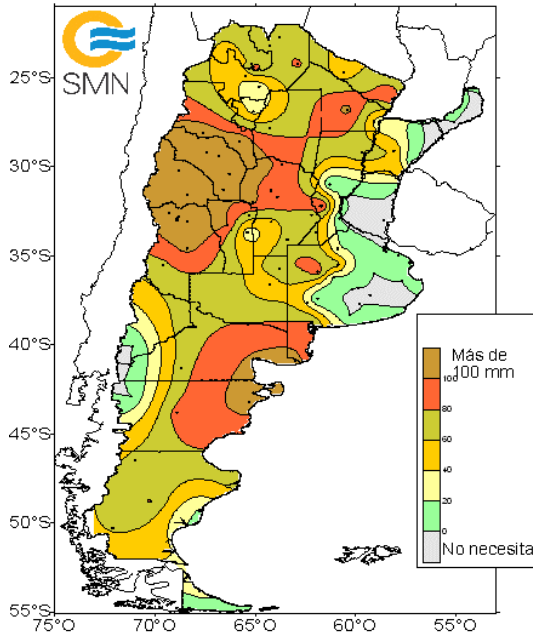
Agua necesaria para no estar en Sequia en los próximos 10 días a partir del 31 de julio de 2023
