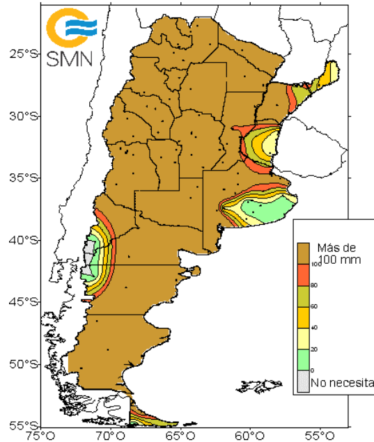
Agua necesaria para comenzar a tener Excesos en los próximos 10 días a partir del 31 de julio de 2023
