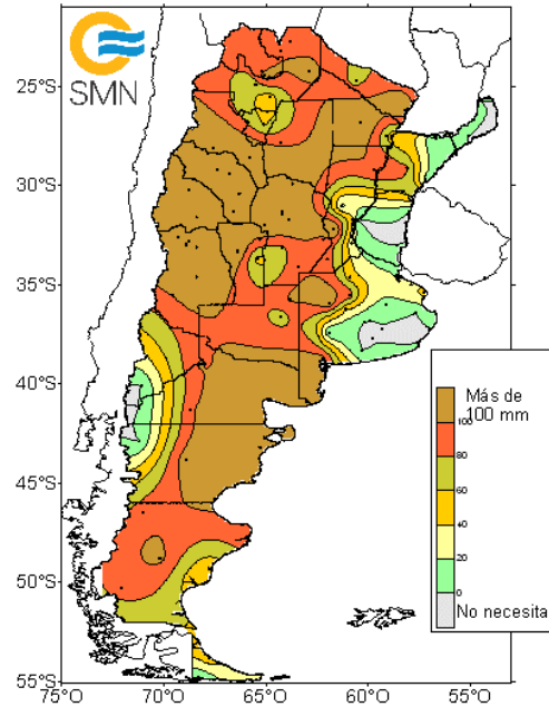
Agua necesaria para no estar en Comienzo de Sequia en los próximos 10 días a partir del 31 de julio de 2023
