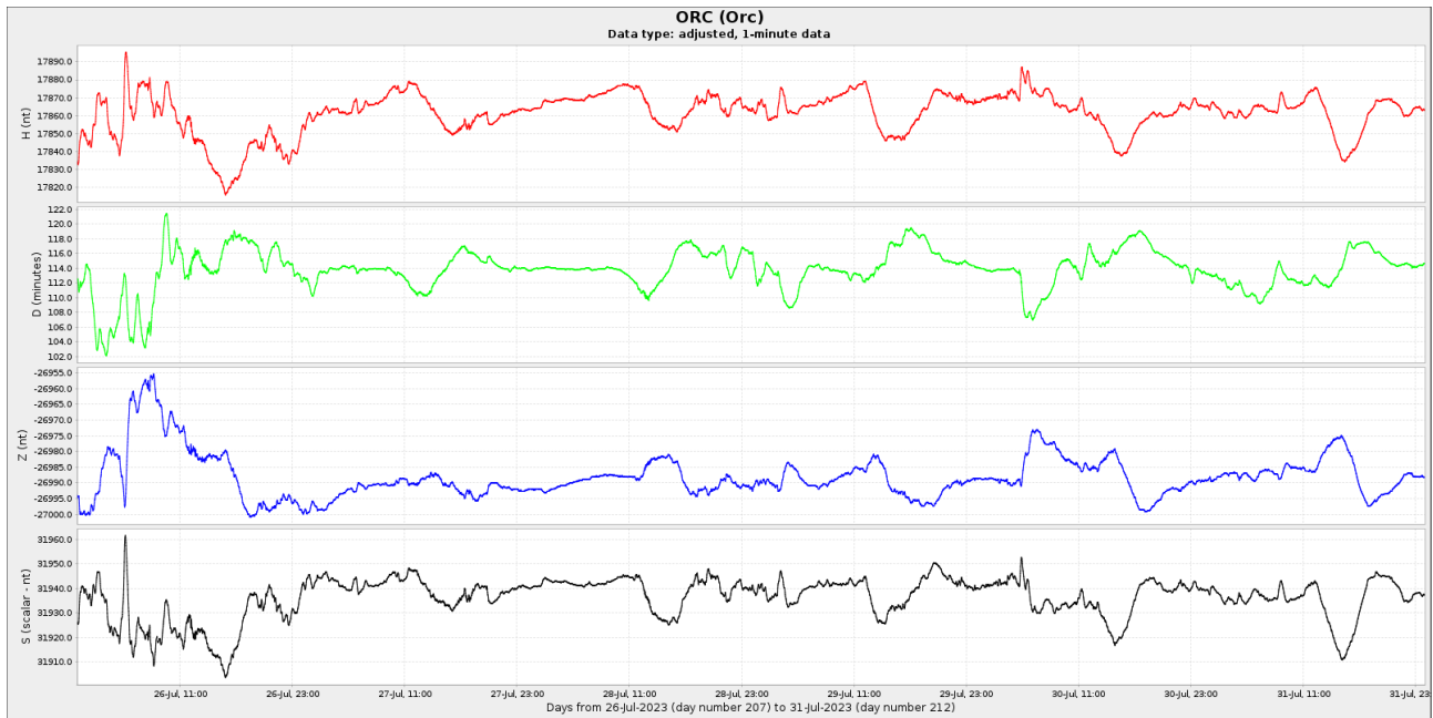
Figura 4c: Componentes del campo magnético del 21 al 30 de julio. En rojo se ve la componente horizontal (H) y en azul la vertical (Z), ambas en nT. En verde se presenta la declinación del campo magnético (D) en minutos y en negro la intensidad del campo magnético en nT.
