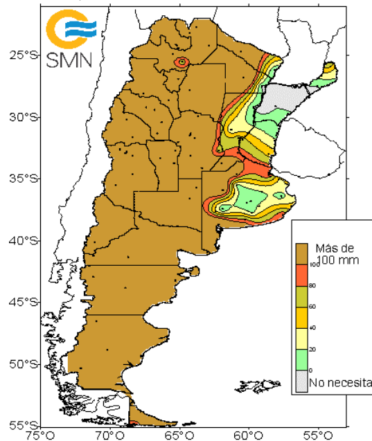
Agua necesaria para comenzar a tener Excesos en los próximos 10 días a partir del 31 de diciembre de 2023
