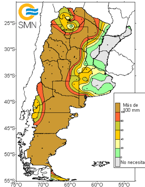
Agua necesaria para no estar en Comienzo de Sequia en los próximos 10 días a partir del 31 de diciembre de 2023
