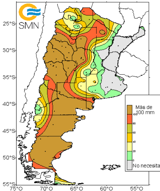
Agua necesaria para no estar en Sequia en los próximos 10 días a partir del 31 de diciembre de 2023
