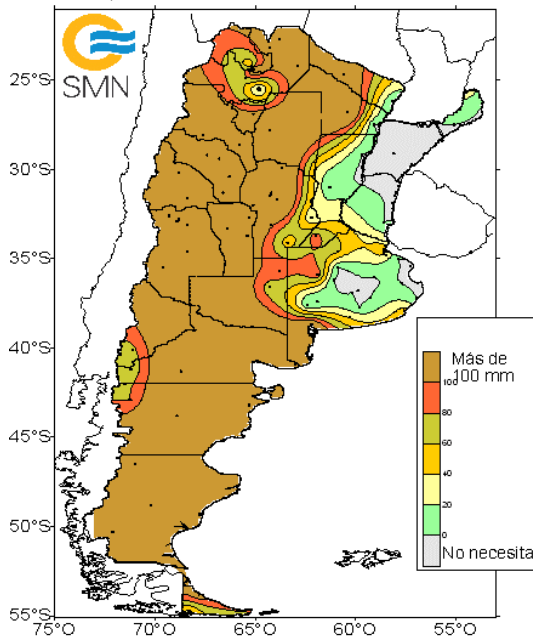
Agua necesaria para tener Buenas Condiciones en los próximos 10 días a partir del 31 de diciembre de 2023
