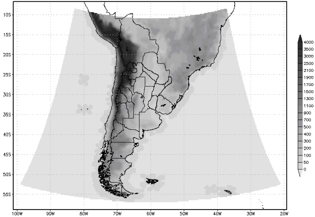
Figura 1. Topografía del dominio utilizado (m).
