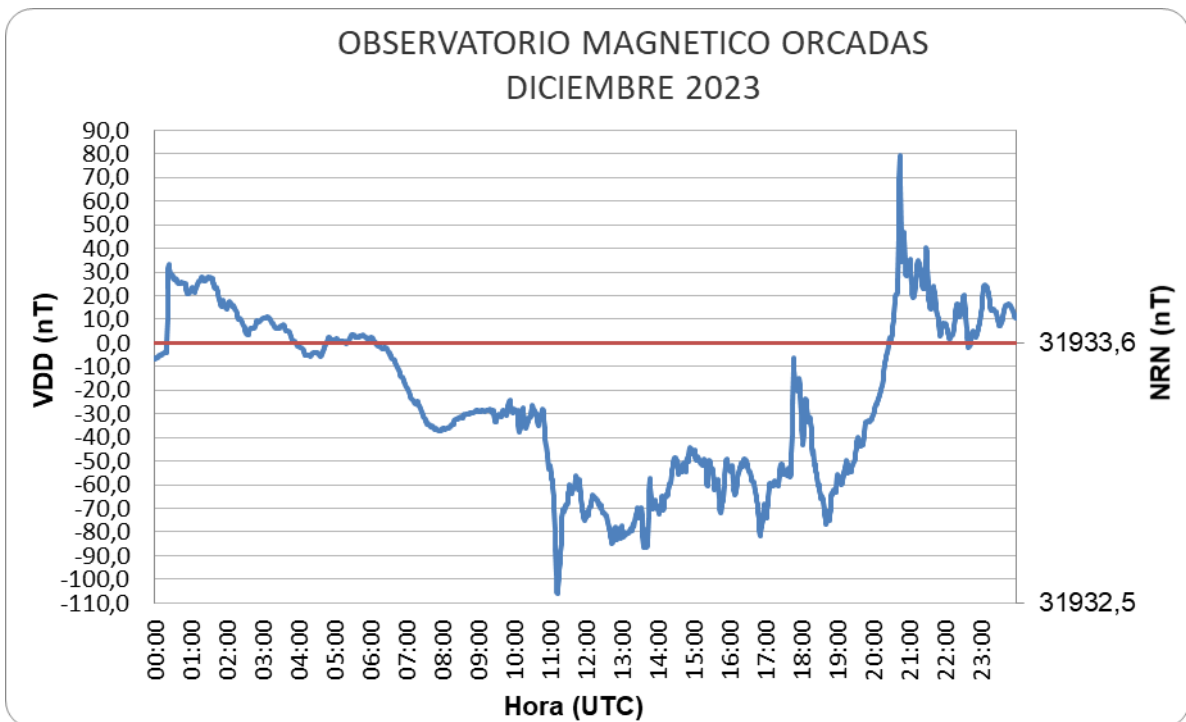
Figura 9: Variación Diaria Perturbada del mes de diciembre
