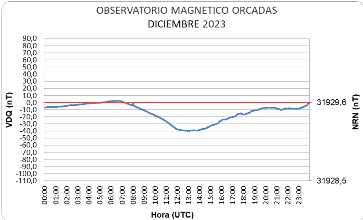
Figura 8: Variación Diaria Calma del mes de diciembre
