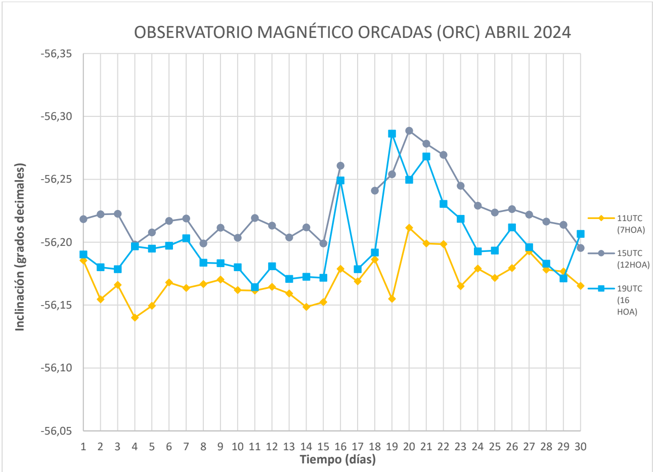
Figura 6: Inclínación magnética en función del tiempo
