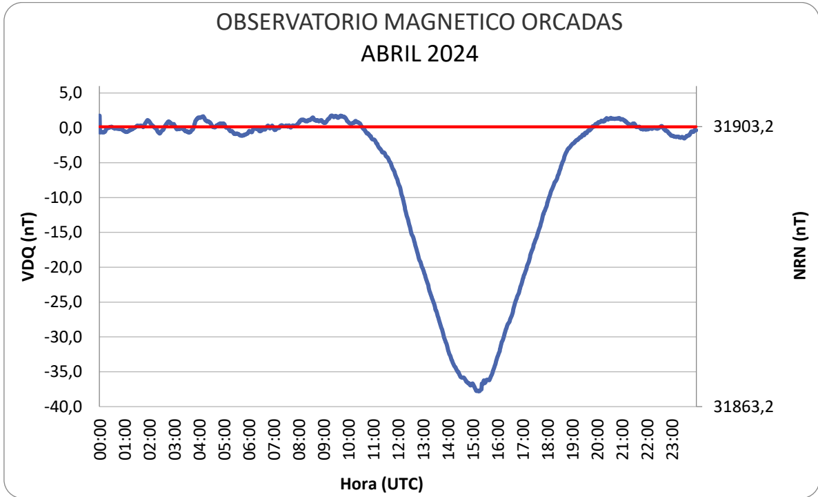
Figura 8: Variación Diaria Calma del mes de abril
