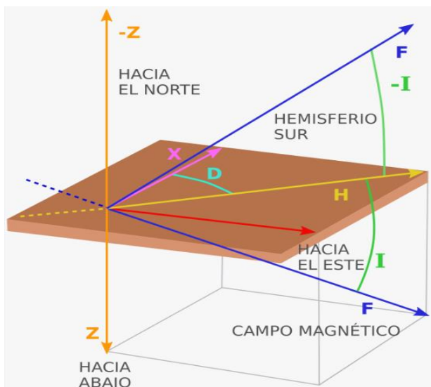
Figura SEQ Figura \* ARABIC 3: Componentes del campo magnético
