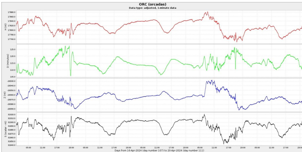
Figura 4b Componentes del campo magnético del 11 al 20 de abril. En rojo se ve la componente horizontal (H) y en azul la vertical (Z), ambas en nT. En verde se presenta la declinación del campo magnético (D) en minutos y en negro la intensidad del campo magnético en nT.
