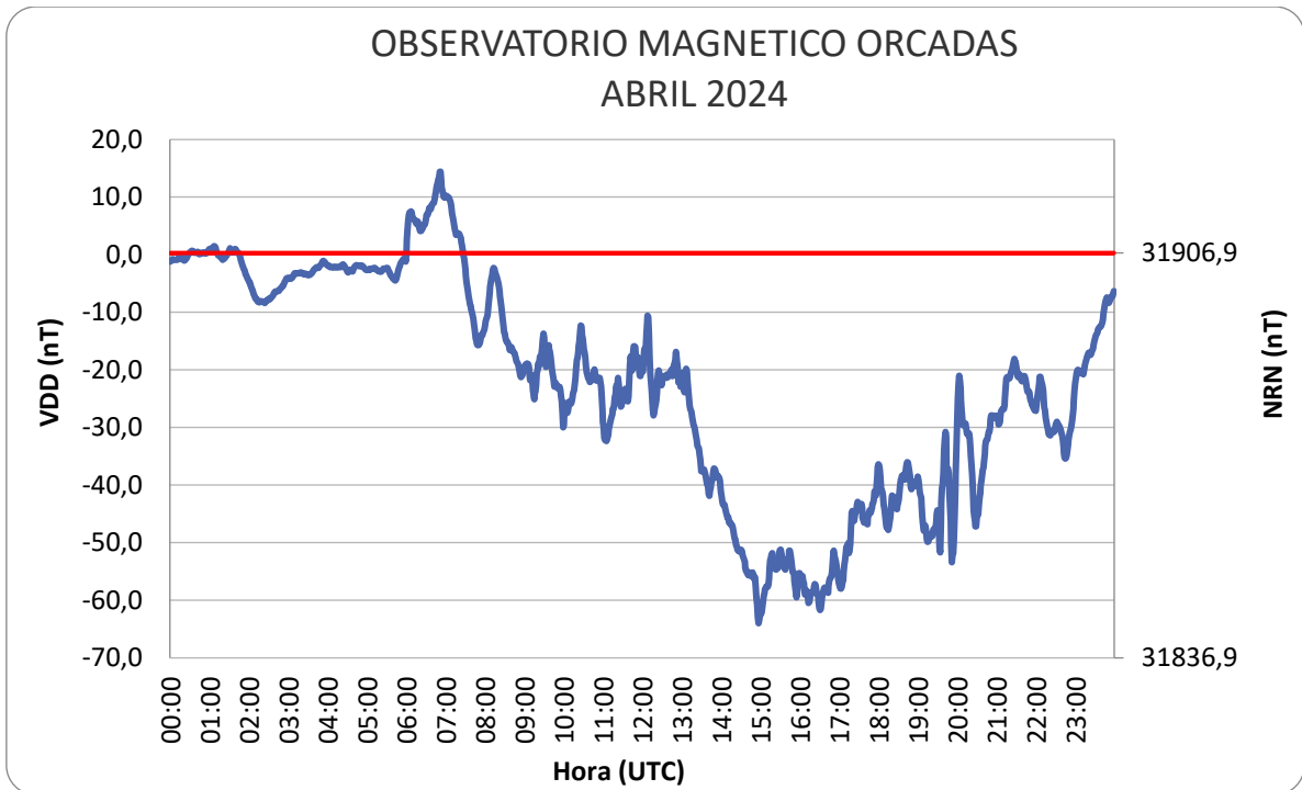
Figura 9: Variación Diaria Perturbada del mes de abril
