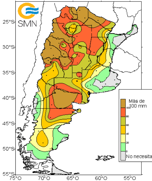
Agua necesaria para no estar en Sequía en los próximos 10 días a partir del 10 de octubre de 2024
