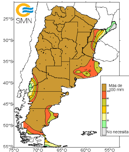
Agua necesaria para comenzar a tener Excesos en los próximos 10 días a partir del 10 de octubre de 2024
