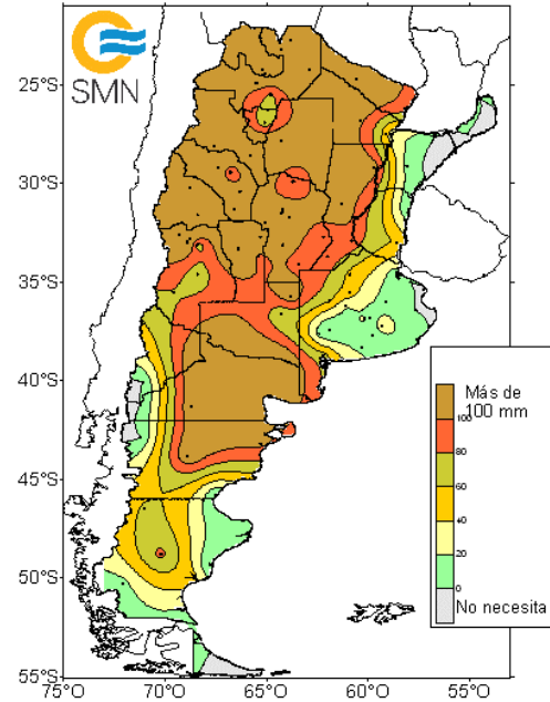
Agua necesaria para no estar en Comienzo de Sequía en los próximos 10 días a partir del 10 de octubre de 2024
