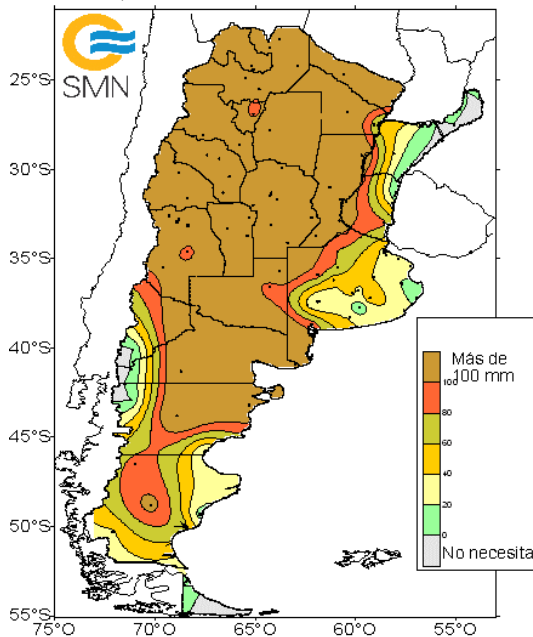
Agua necesaria para tener Buenas Condiciones en los próximos 10 días a partir del 10 de octubre de 2024
