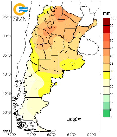
Evapotranspiración Potencial Década al 20 de octubre de 2024
