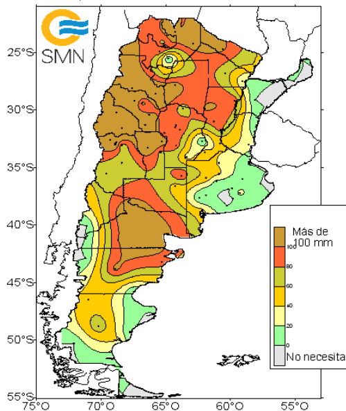
Agua necesaria para no estar en Sequía en los próximos 10 días a partir del 20 de octubre de 2024
