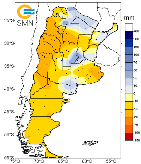
Diferencia entre Precipitación y ETP Década al 20 de octubre de 2024
