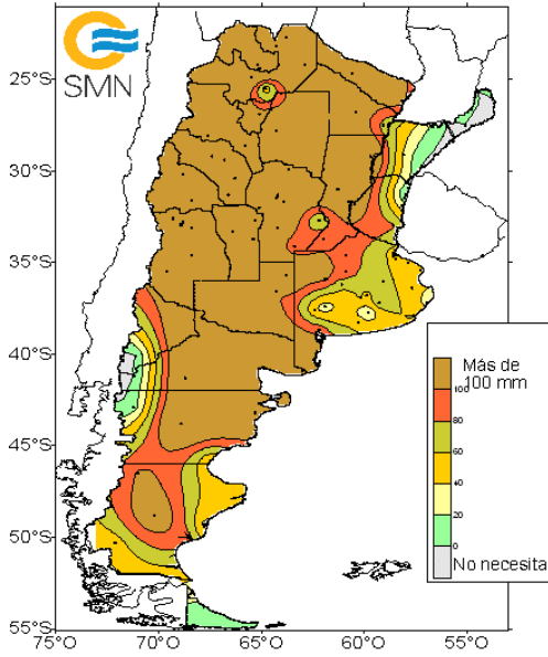
Agua necesaria para tener Buenas Condiciones en los próximos 10 días a partir del 20 de octubre de 2024
