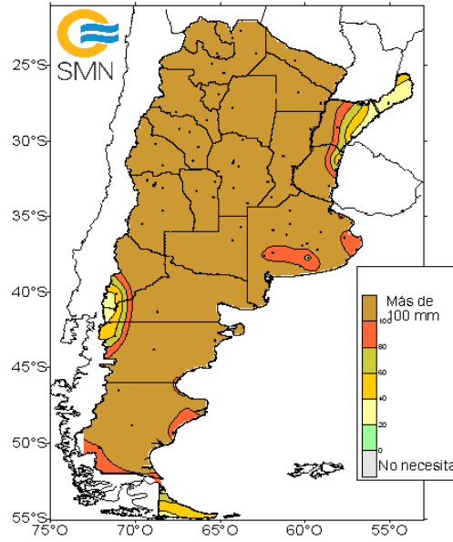
Agua necesaria para comenzar a tener Excesos en los próximos 10 días a partir del 20 de octubre de 2024
