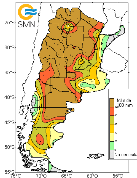
Agua necesaria para no estar en Comienzo de Sequía en los próximos 10 días a partir del 20 de octubre de 2024
