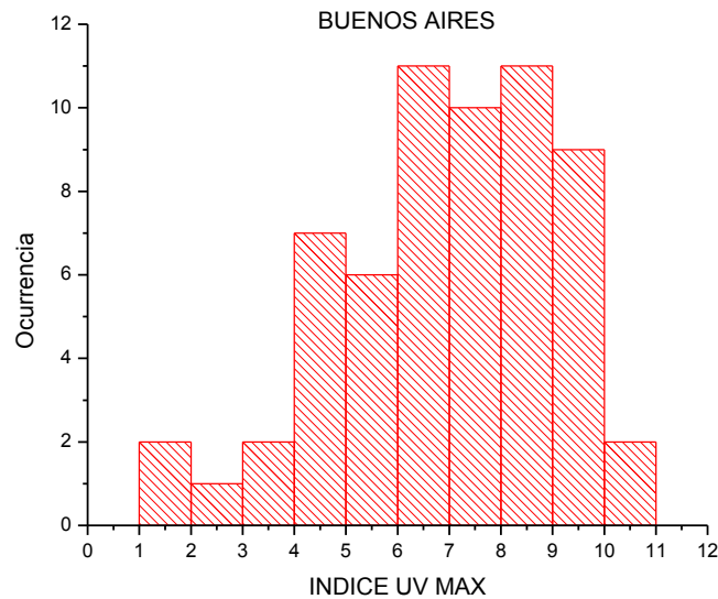
Figura 13. Histograma con los valores de índice UV máximo diario medidos en Buenos Aires.
