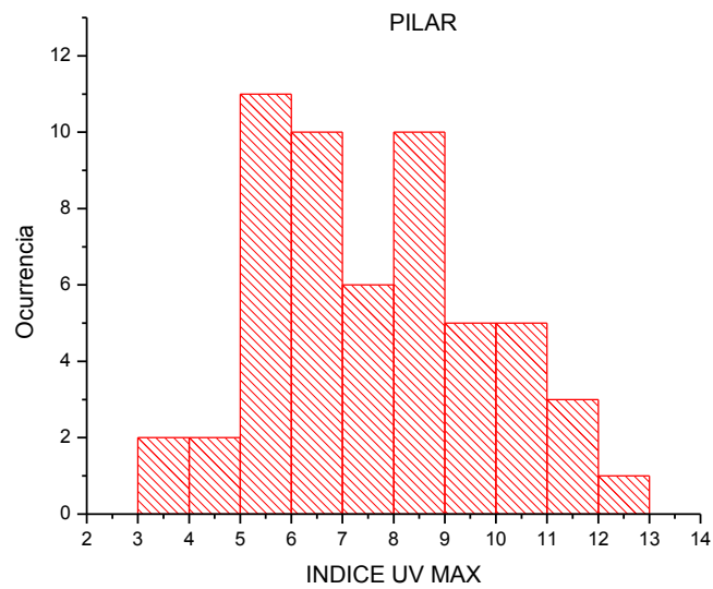
Figura 12. Histograma con los valores de índice UV máximo diario medidos en Pilar.
