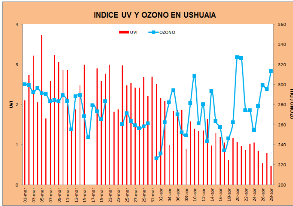
Figura 16. Columna total de ozono medida en Ushuaia.
