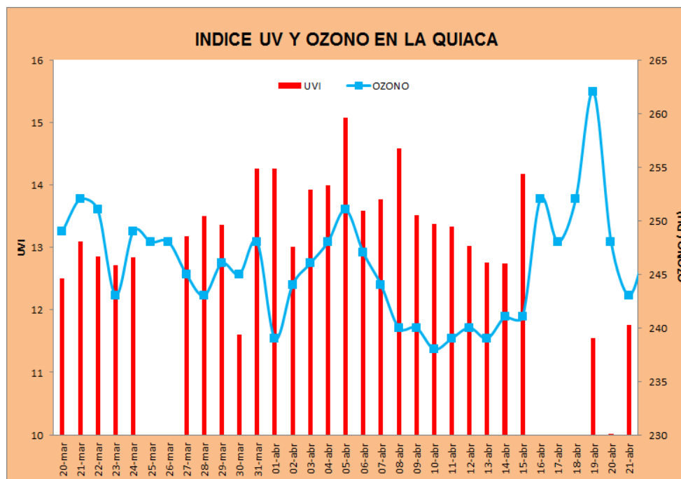
Figura 18. Columna total de ozono medida en La Quiaca.
