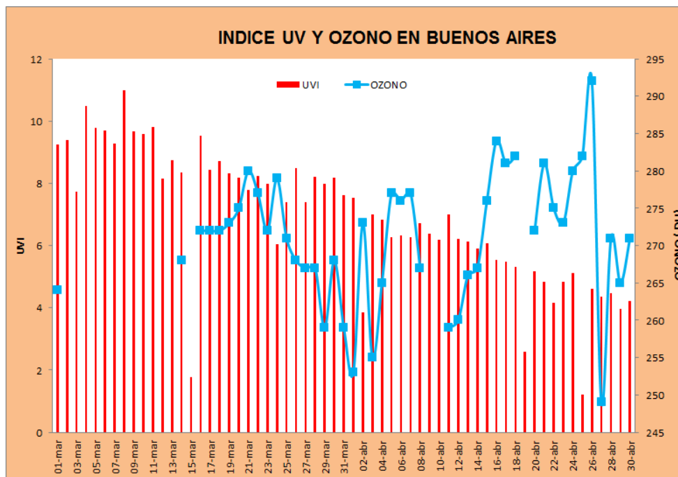
Figura 15. Columna total de ozono medida en Buenos Aires.
