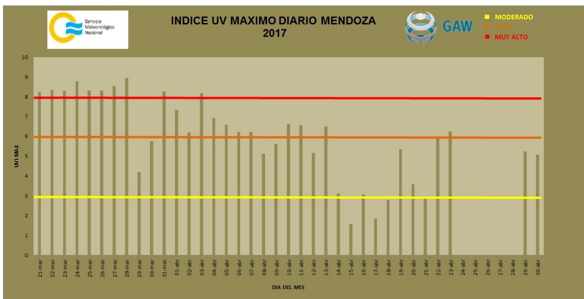
Figura 8. Índice UV máximo diario medido en Mendoza.
