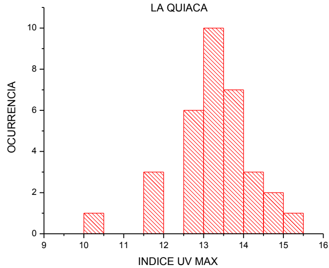
Figura 11. Histograma con los valores de índice UV máximo diario medidos en La Quiaca.
