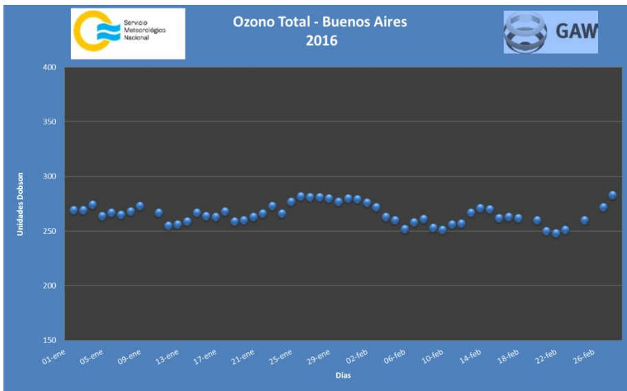
Figura 7. Columna total de ozono medida en Buenos Aires.
