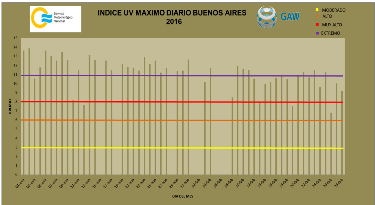
Figura 4. Índice UV máximo diario medido en Buenos Aires.
