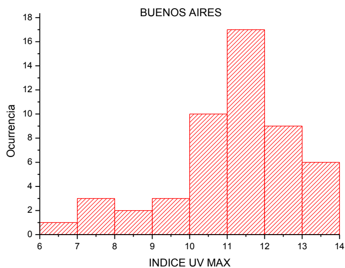
Figura 6. Histograma con los valores de índice UV máximo diario medido en Buenos Aires
