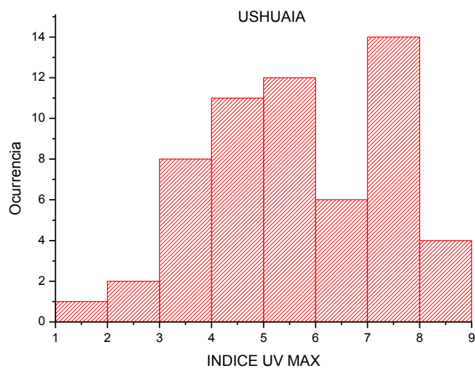
Figura 5. Histograma con los valores de índice UV máximo diario medido en Ushuaia
