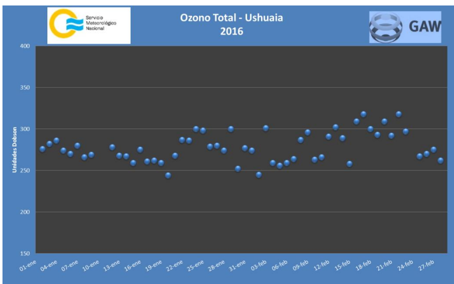
Figura 8. Columna total de ozono medida en Ushuaia.
