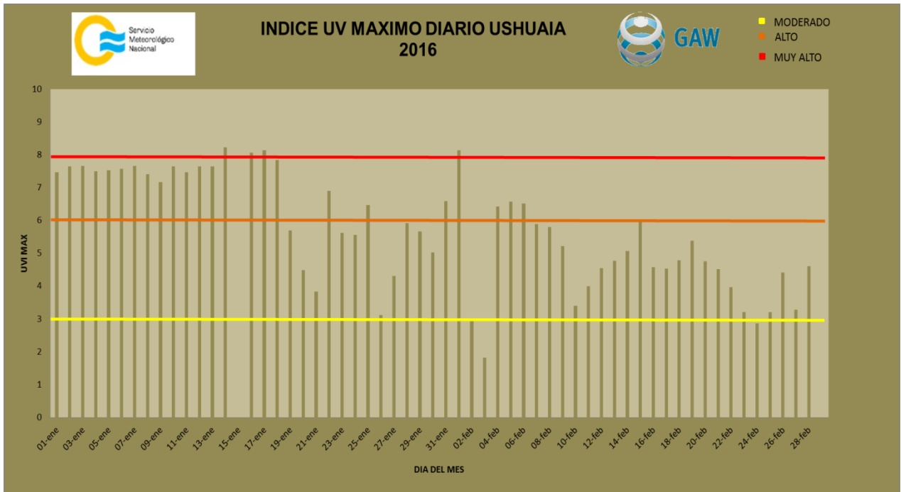
Figura 3. Índice UV máximo diario medido en Ushuaia
