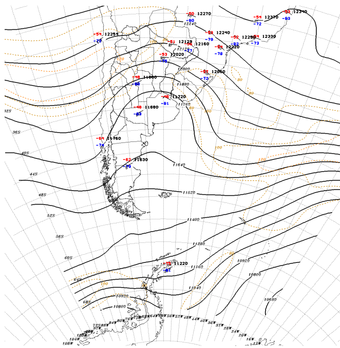
ANÁLISIS GEOP. E ISOTACAS EN 200hPA DEL 2014/08/25 A LAS 12 Z-SHJ Figura 8: Geopotencial (mgp) e isotacas (kt) en 200 hPa para el 25 de Agosto de 2014 a las 12 UTC
