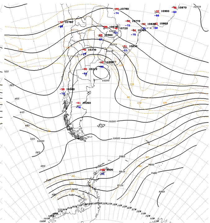
ANÁLISIS GEOP. E ISOTACAS EN 250hPA DEL 2014/08/25 A LAS 12 Z-SHJ Figura 7: Geopotencial (mgp) e isotacas (kt) en 250 hPa para el 25 de Agosto de 2014 a las 12 UTC
