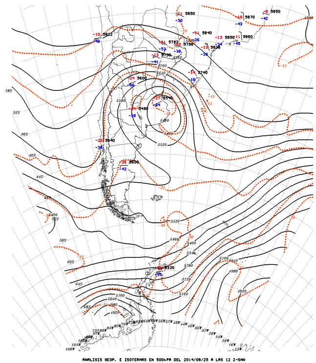
Figura 5: Geopotencial (mgp) e isotermas (kt) en 500 hPa para el 25 de Agosto de 2014 a las 12 UTC
