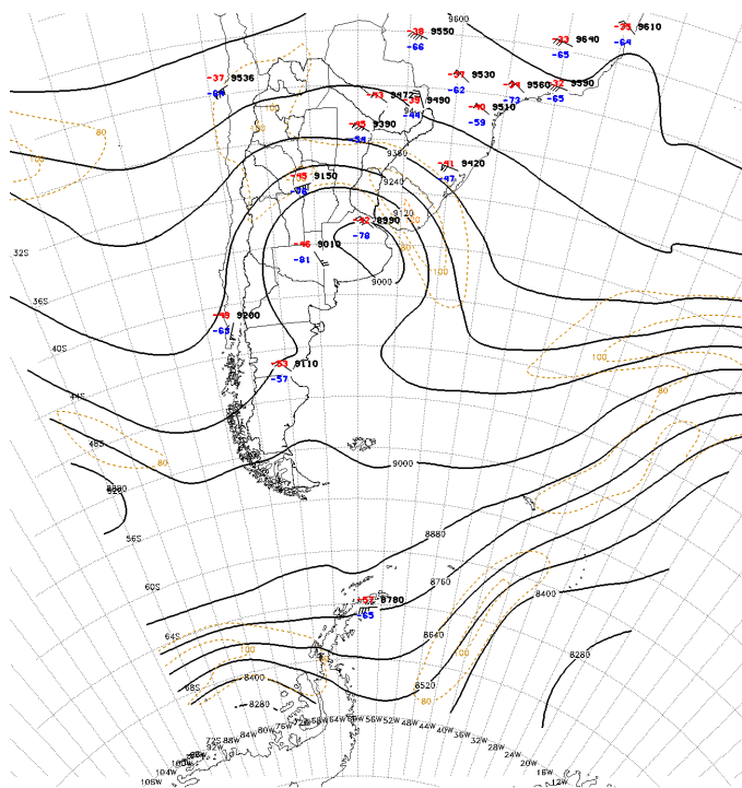
ANÁLISIS GEOP. E ISOTACAS EN 300hPA DEL 2014/08/25 A LAS 12 Z-SHJ Figura 6: Geopotencial (mgp) e isotacas (kt) en 300 hPa para el 25 de Agosto de 2014 a las 12 UTC
