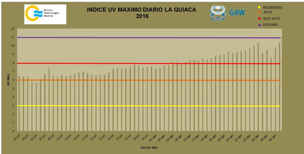
Figura 4. Índice UV máximo diario medido en La Quiaca.
