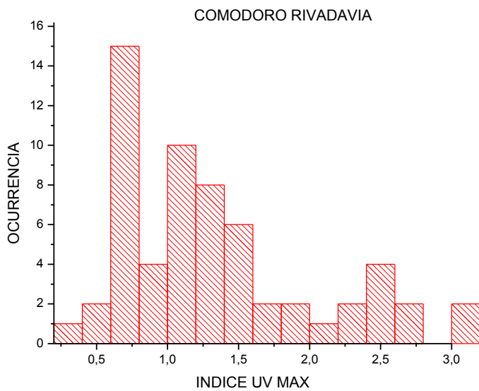
Figura 10. Histograma con los valores de índice UV máximo diario medidos en Comodoro Rivadavia.
