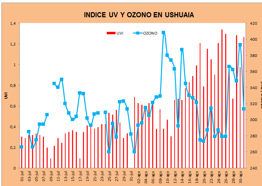
Figura 16. Columna total de ozono medida en Ushuaia.
