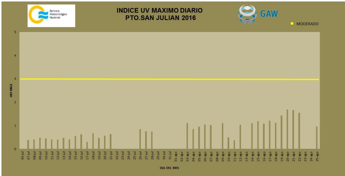
Figura 7. Índice UV máximo diario medido en Pto. San Julian.
