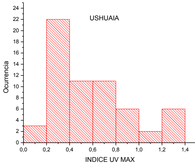
Figura 9. Histograma con los valores de índice UV máximo diario medidos en Ushuaia
