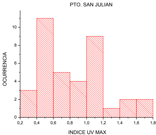
Figura 13. Histograma con los valores de índice UV máximo diario medidos en Pto. San Julian.
