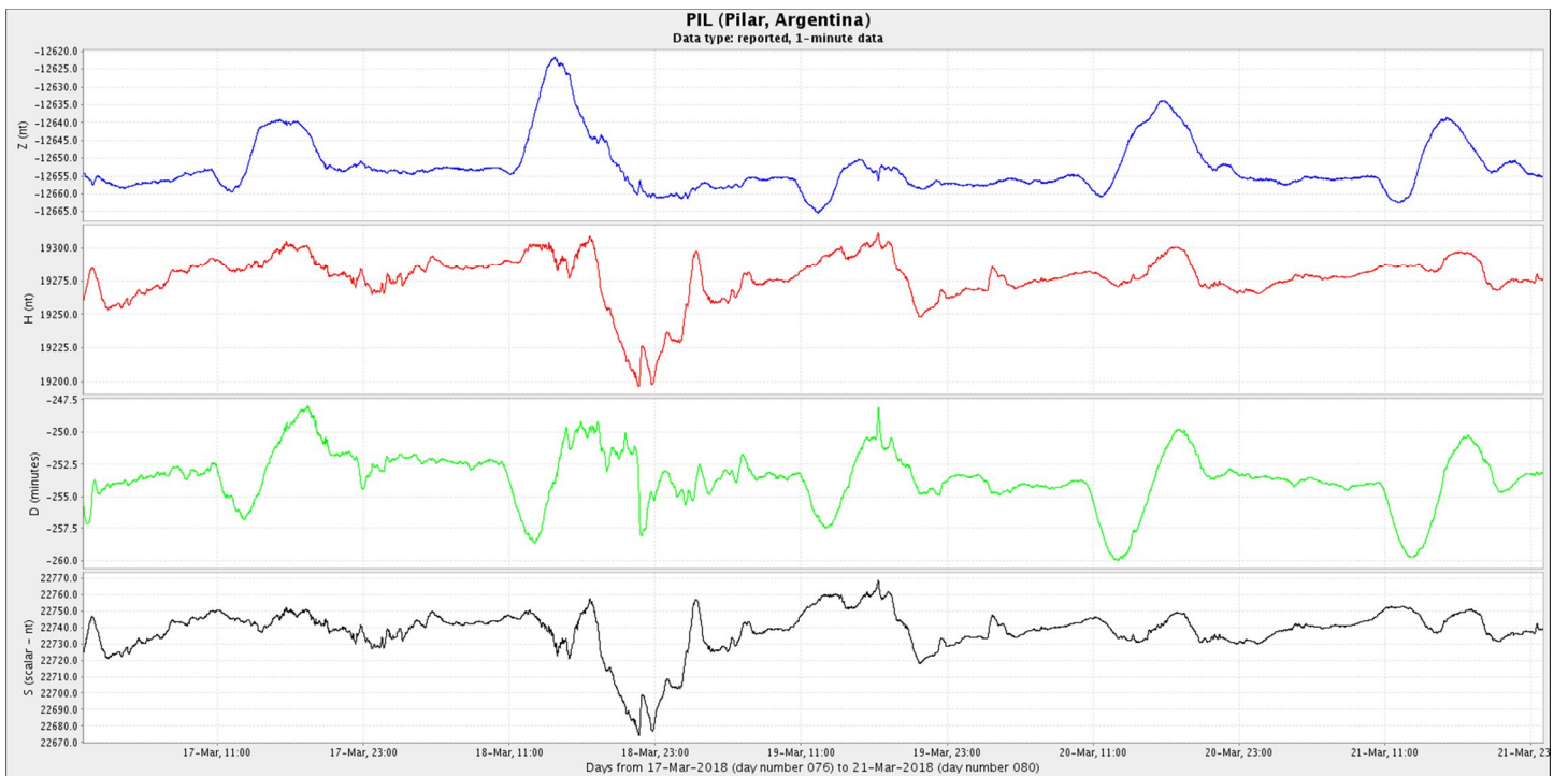
Figura 4b: Componentes del campo magnético del 11 al 21 de marzo. En rojo se ve la componente horizontal (H) y en azul la vertical (Z), ambas en nT. En verde se presenta la declinación del campo magnético (D) en minutos y en negro la intensidad del campo magnético en nT.
