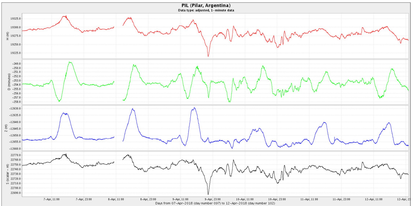
Figura 4a: Componentes del campo magnético del 1 al 12 de Abril. En rojo se ve la componente horizontal ( H ) y en azul la vertical ( Z ), ambas en nT. En verde se presenta la declinación del campo magnético ( D ) en minutos y en negro la intensidad del campo magnético en nT
