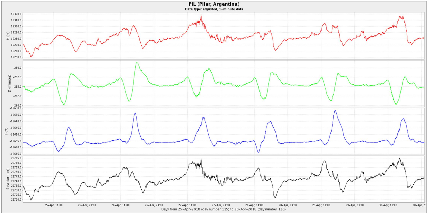
Figura 4c: Componentes del campo magnético del 25 al 30 de Abril. En rojo se ve la componente horizontal (H) y en azul la vertical (Z), ambas en nT. En verde se presenta la declinación del campo magnético (D) en minutos y en negro la intensidad del campo magnético en nT.
