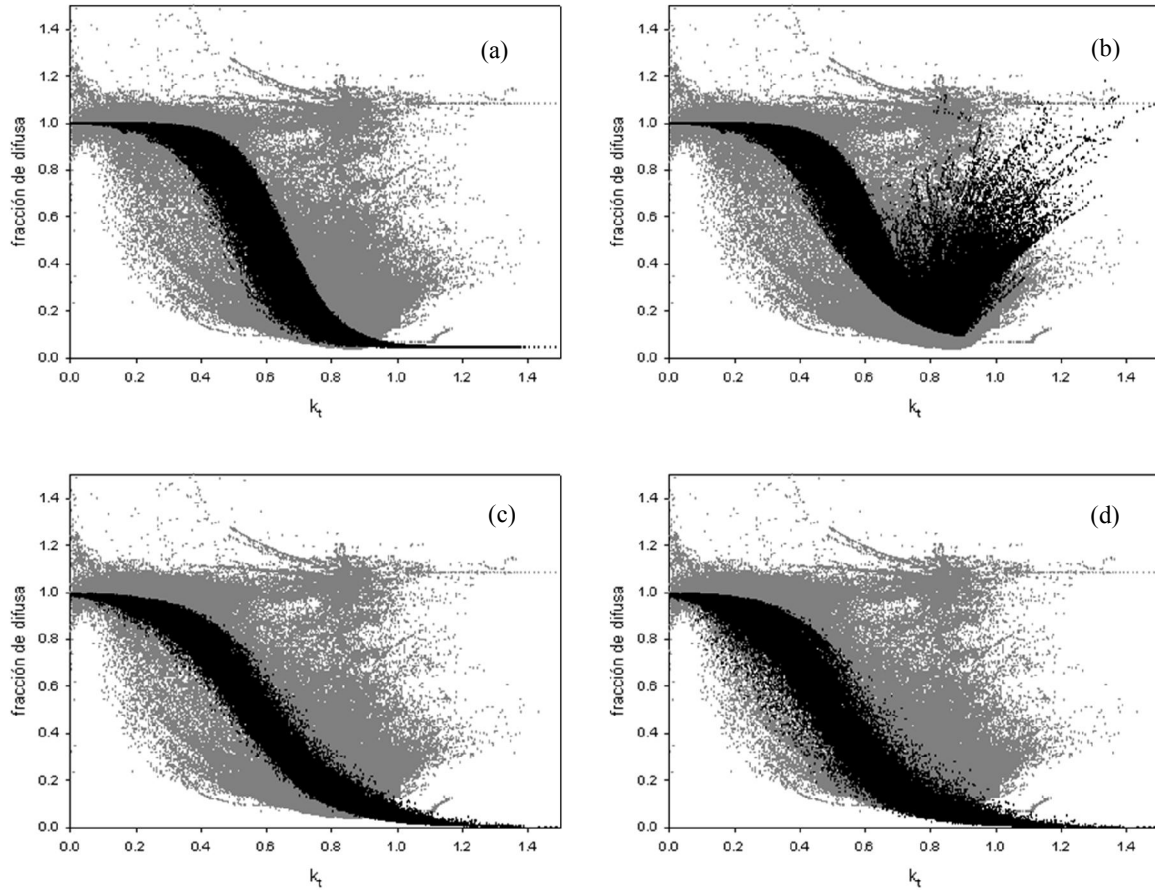
Figura 4. Índice de claridad k_t vs fracción de difusa k_d . Los puntos grises corresponden a los valores medidos de la base de datos completa. Los puntos negros corresponden a los valores de I_D estimados usando los modelos de (a) Eng1, (b) Eng2, (c) BRL, (d) BRL-BR.
