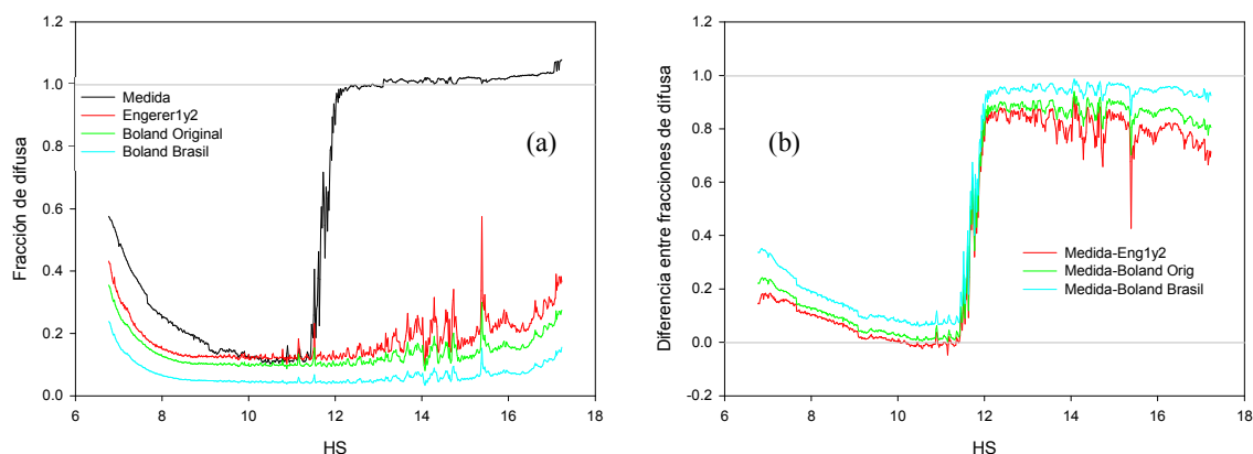
Figura 3. (a) Fracciones de difusa medida y estimadas con Eng1y2, BRL y BRL-BR para el día 243 de 2005. Se observa que la fracción de difusa medida (línea negra) alcanza el valor 1 luego del mediodía, mientras que las estimadas usando los demás modelos no lo hacen. (b) Diferencias de las fracciones de difusa medida vs. estimadas. Se observa que la diferencia para los momentos de desalineación corresponde a valores próximos a 1.
