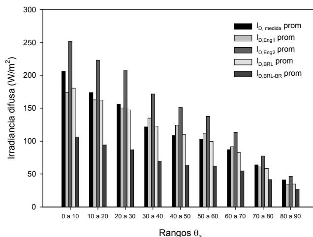
Figura 8. Valores promedios de irradiancia difusa medida y estimada según cada modelo, para rangos de ángulo cenital de tamaño 10°.
