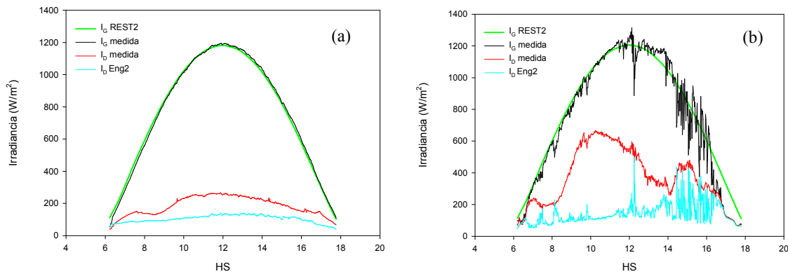
Figura 1. Valores medidos de Irradiancia solar global I_G y difusa I_D , y valores estimados de Irradiancia solar global de día claro (usando el modelo REST2) y de difusa usando el modelo de Eng2 para los días (a) día 295 de 2005 y (b) día 298 de 2005. HS es hora solar.
