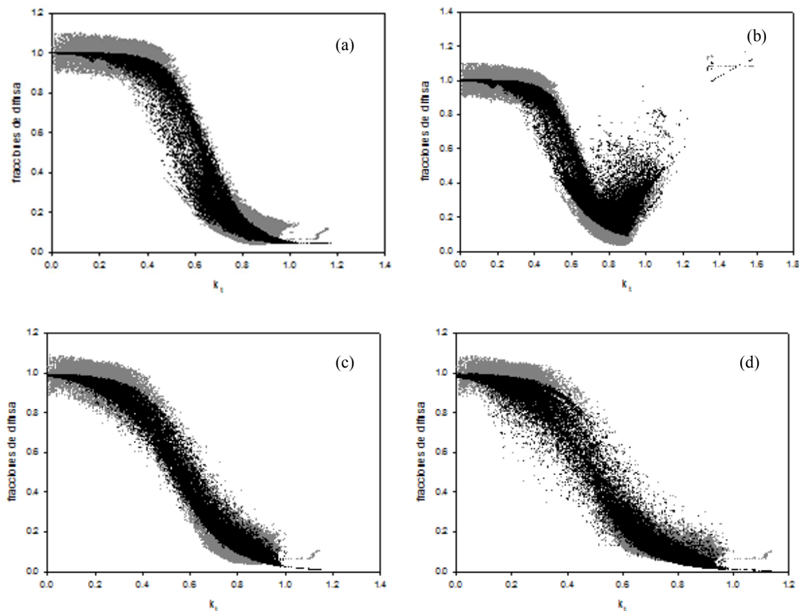
Figura 6. Índice de claridad k_t vs fracción de difusa k_d . Los puntos grises corresponden a los valores medidos de la base de datos filtrada. Los puntos negros corresponden a los valores de I_D estimados usando los modelos de (a) Eng1, (b) Eng2, (c) BRL, (d) BRL-BR.
